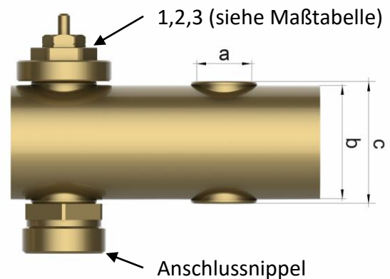
Abb. 1 vertikales Stichmaß eines Verteilerbalkens
